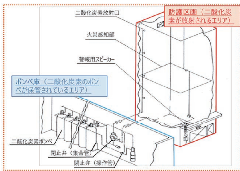
現行の二酸化炭素消火設備の構成例
