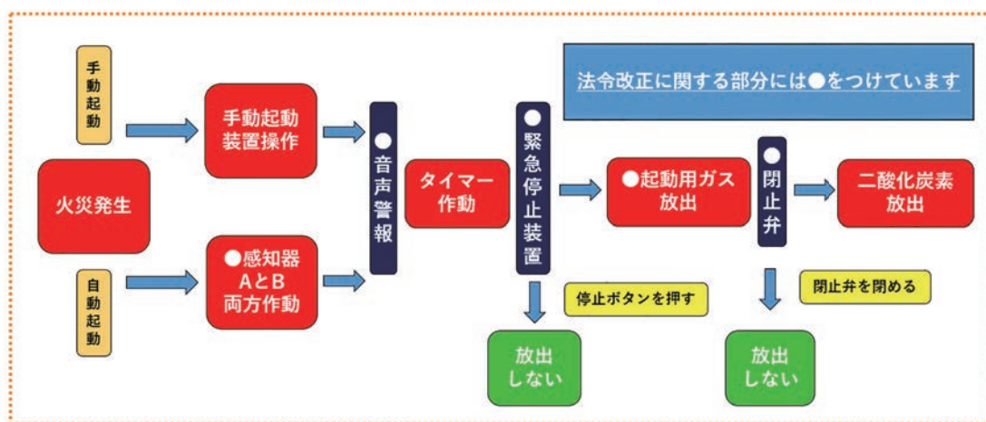
現行の作動フロチャート例
